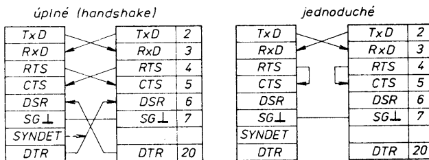
Obr. 1. Vzájemné propojení pomocí RS232C
